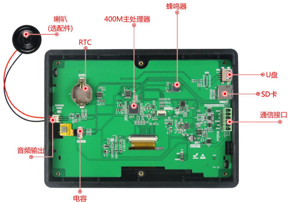
图 1-2 硬件配置图
